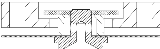
Fig. 14.3.3 "ASSEMBLAGE DETAILS (32) ET (35)"
