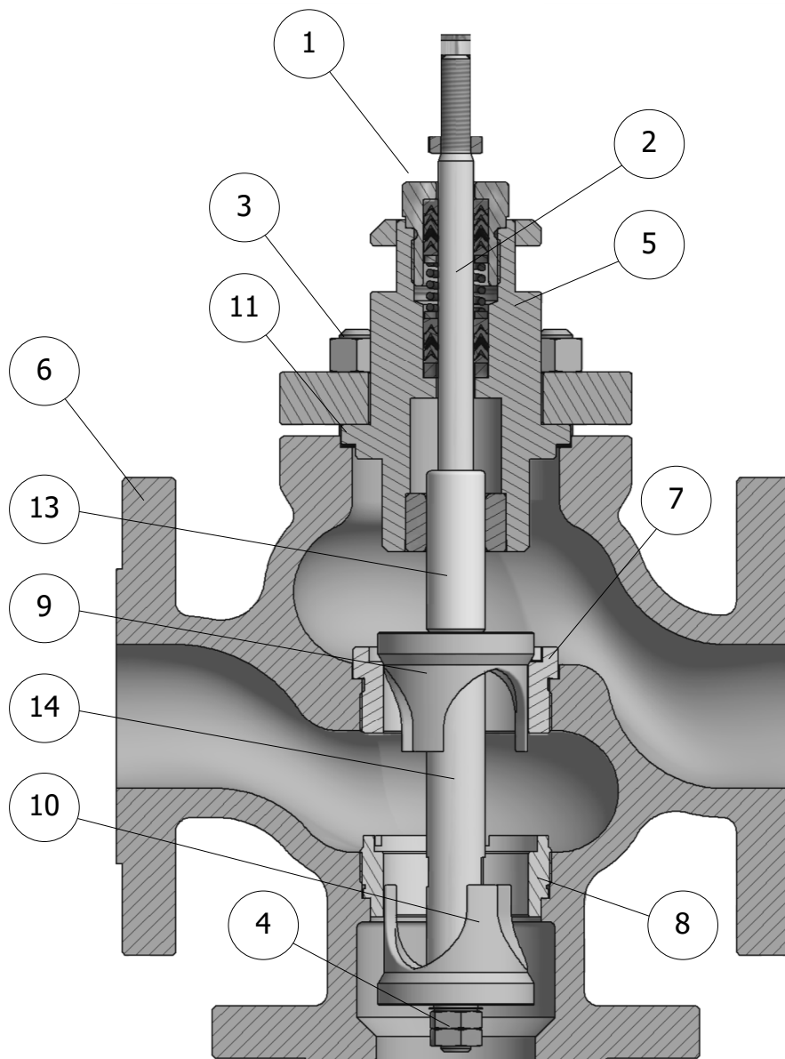
Fig. 7 Vanne de dérivation
