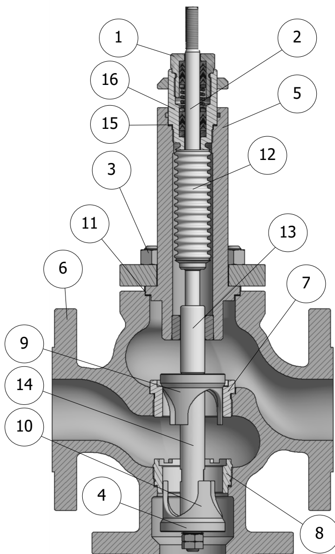
Fig. 9 Vanne de dérivation avec soufflet
