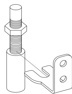
Fig. 4.3.3 Valve spindle adaptor 180-23 Adattatore perno di feedback 180-23
