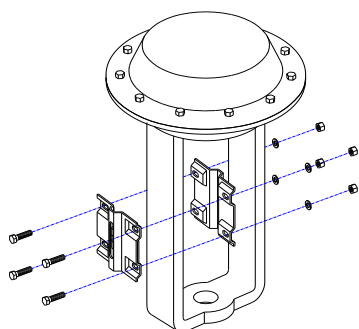
Fig. 4.3.1 Fixing kit 072-55 Kit di fissaggio 072-55
