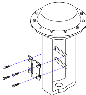
Fig. 4.3.2 Fixing kit 973SUP Kit di fissaggio 973SUP
