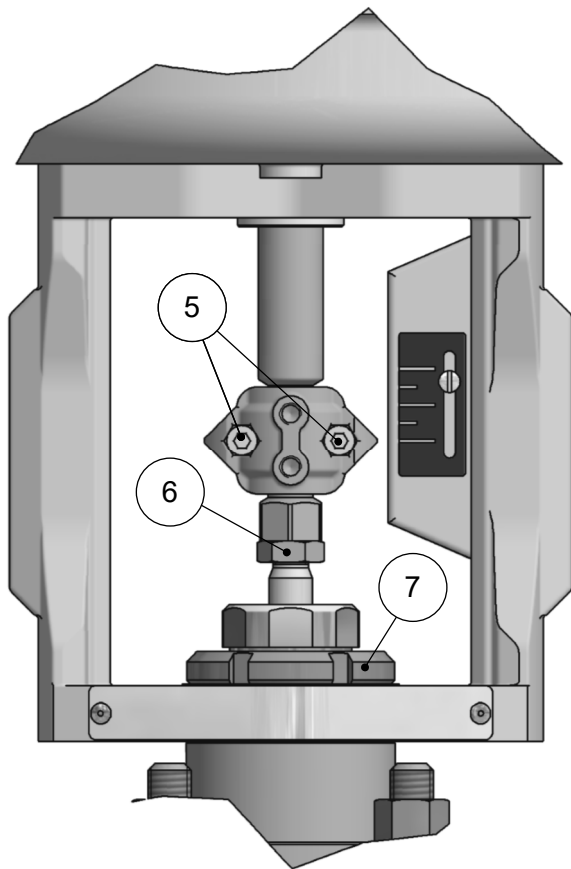
Fig. 17 Válvulas 1/2" ÷ 2"
