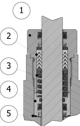
Fig. 13 «SP400»
