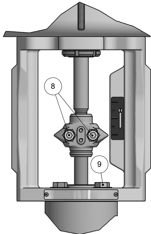
Fig. 18 Válvulas 3" ÷ 4"
