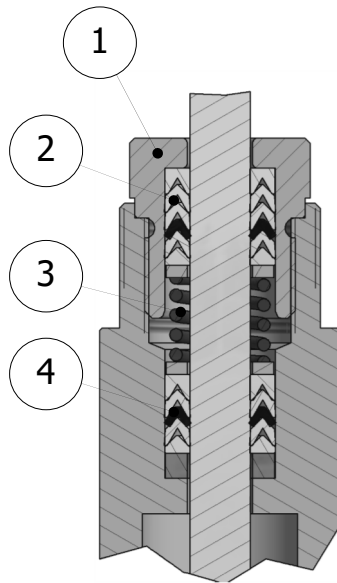
Fig. 9 «SP200»
